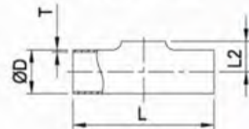
DIN PT 等径平口三通
