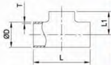
变径短三通
