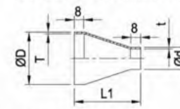
SMS ER 偏心大小头 SMS ER SMS Eccentric Reducer
