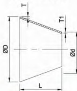
DIN CR 同心大小头
