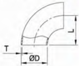
DIN 90° Short Bend
