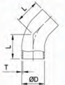
45° long elbow
