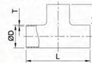
短三通
