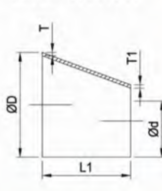
DIN ER 偏心大小头
