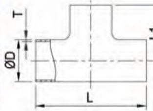
Long Tee
