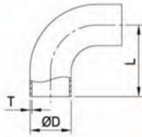
90° Long Bend
