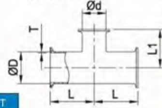
夹式三通 C.7MP-Clamp Long Tee
